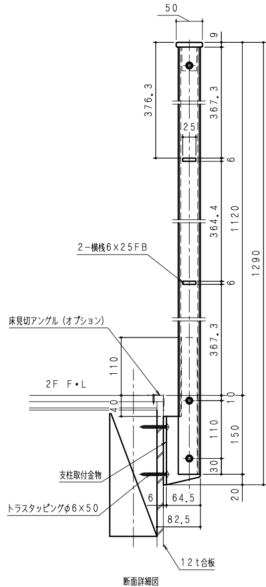
断面詳細図
