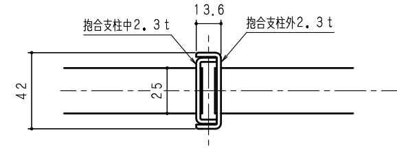
A-A断面 (S=1/2)
