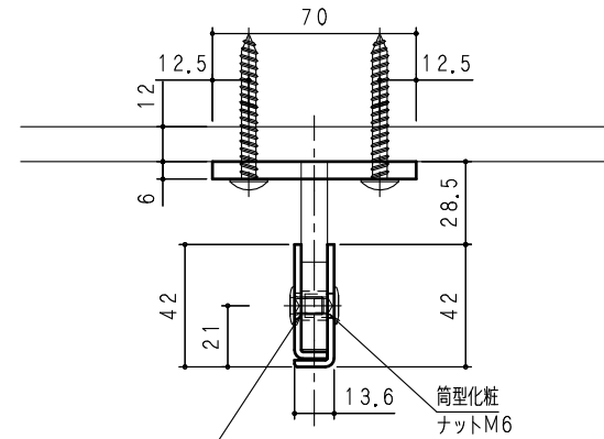
B-B断面 (S=1/2) トルクス化粧平ボルト M6×10
